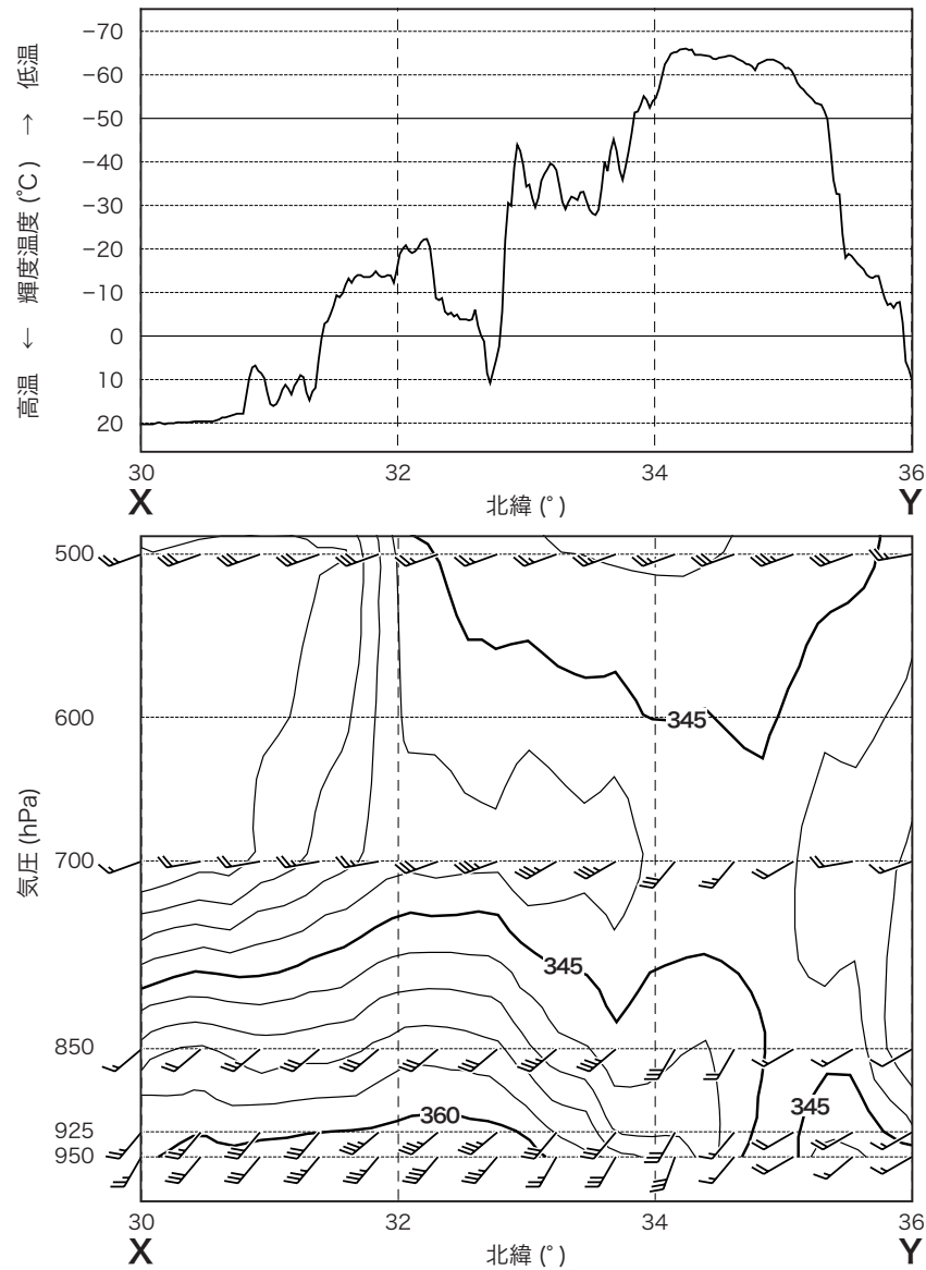
図 12 気象衛星赤外画像の輝度温度 (上), 相当温位・風の鉛直断面図 (下)
