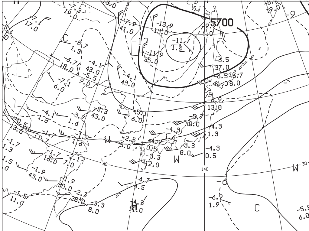
図 3 500hPa 天気図
