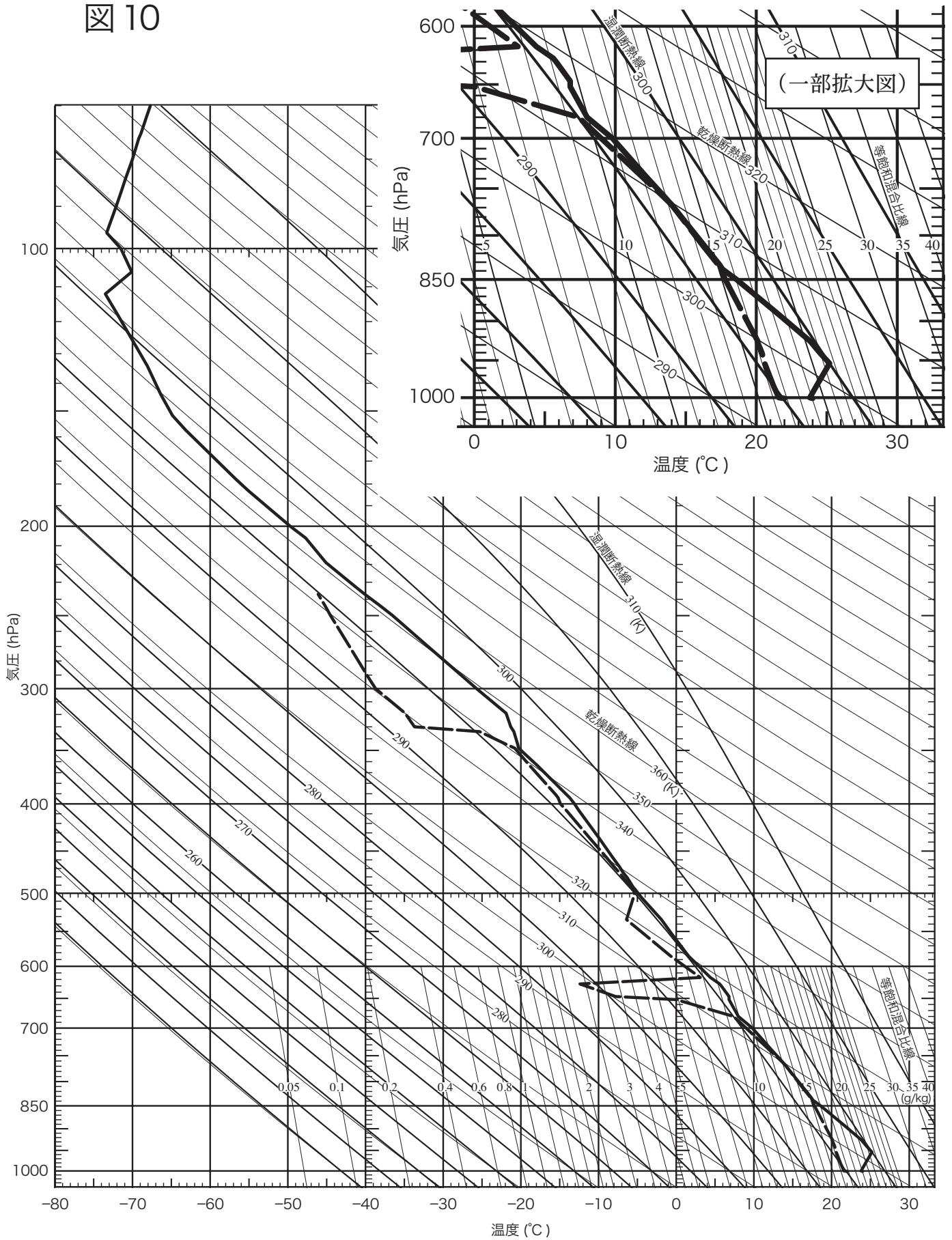
図 10 福岡の状態曲線
