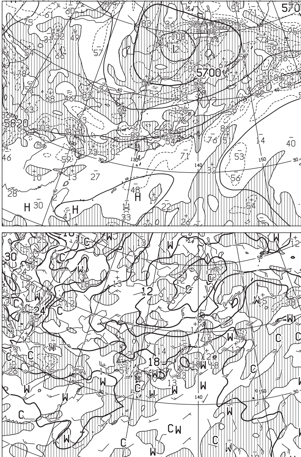
図5 500hPa 高度・渦度解析図 (上)
