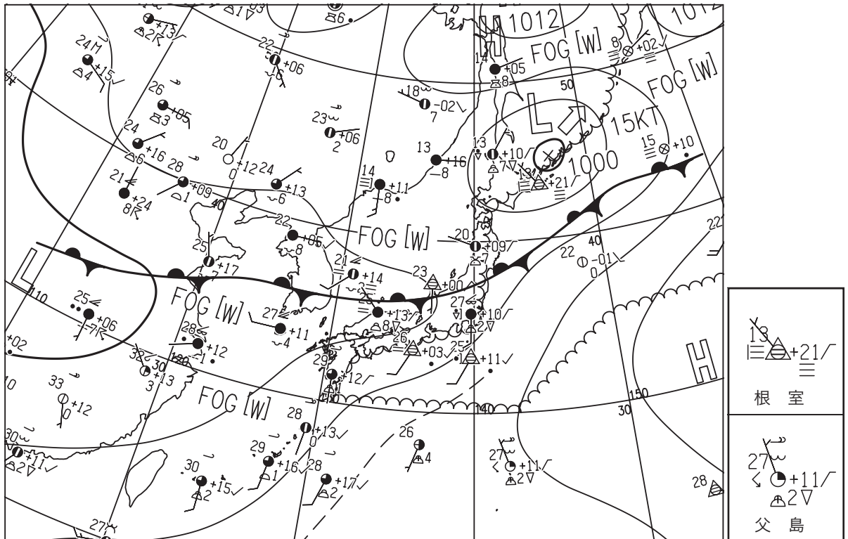
図 1 地上天気図
