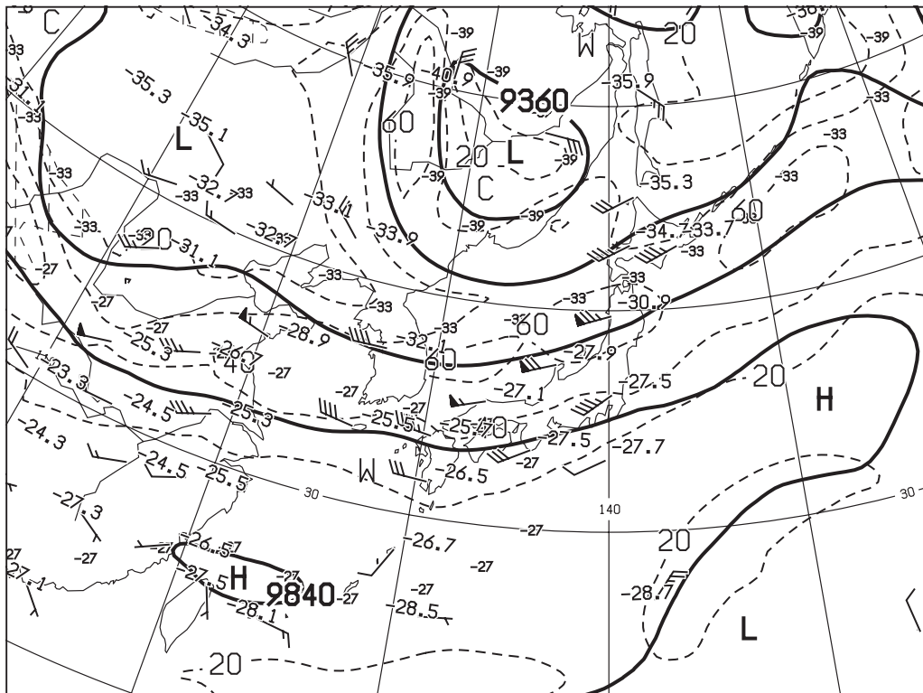
図 2 300hPa 天気図
