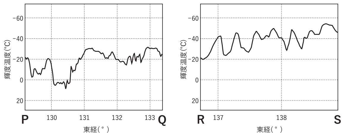
図 8 輝度温度図 図 7 の PQ 間(左), RS 間(右) ※P, Q, R, S の位置は図 7 に表示 XX 年 2 月 26 日 15 時(06UTC)
