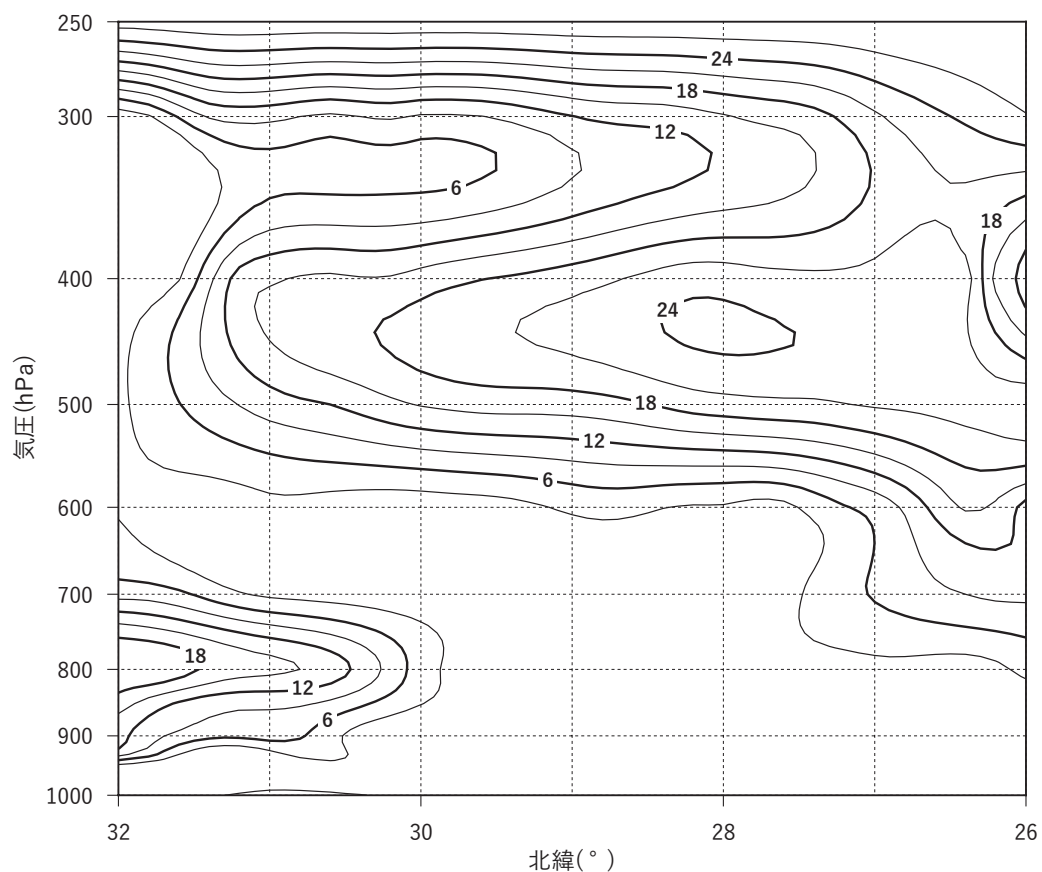
図 9 東経 126° 線上の北緯 26° ~ 32° の湿数鉛直断面図 実線：湿数(°C) XX 年 2 月 26 日 15 時(06UTC)
